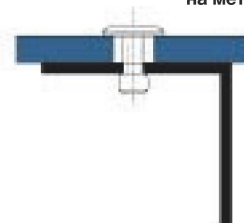
Видиме кріплення заклепками на металевому підрамнику
